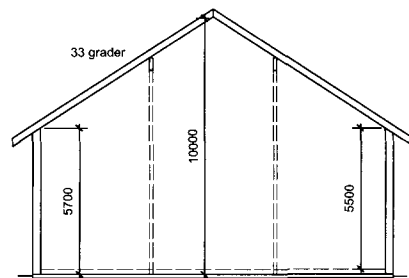
Typisk snitt
