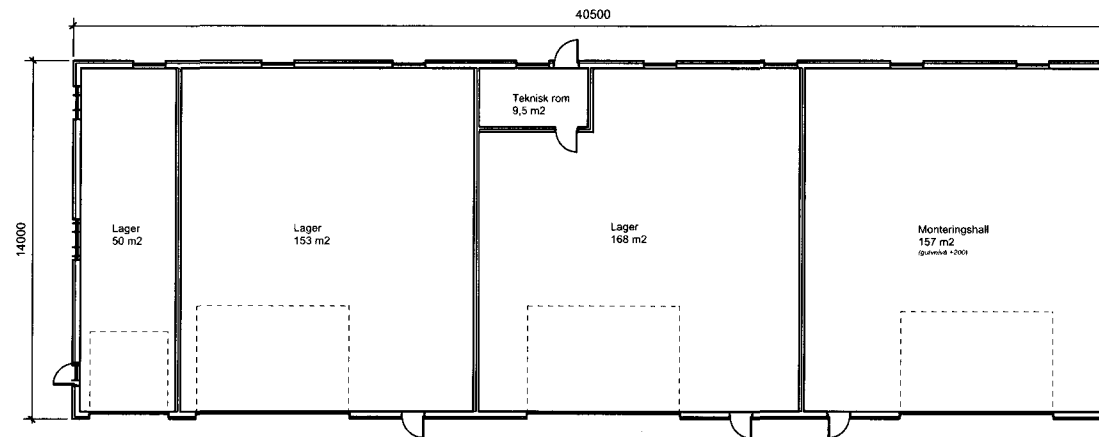
Plan 1. etasje
